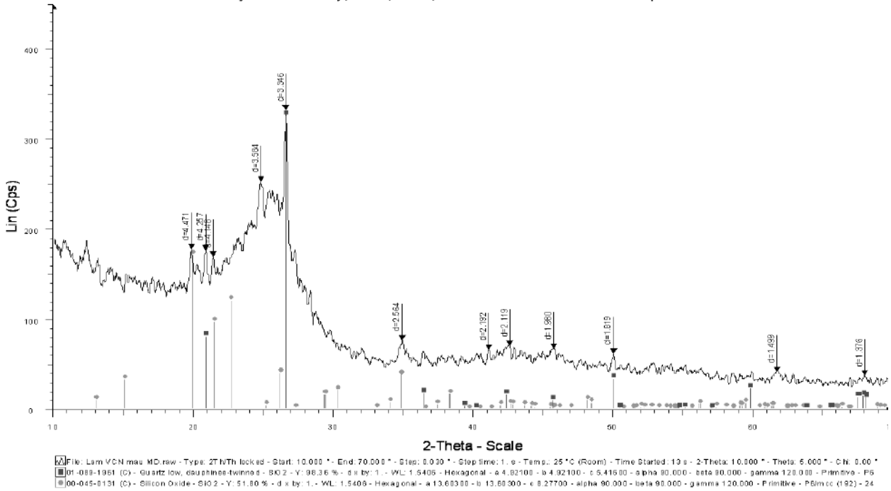
Hình 5: Giản đồ nhiễu xạ tia X của mẫu than mỏ Mông Dương
