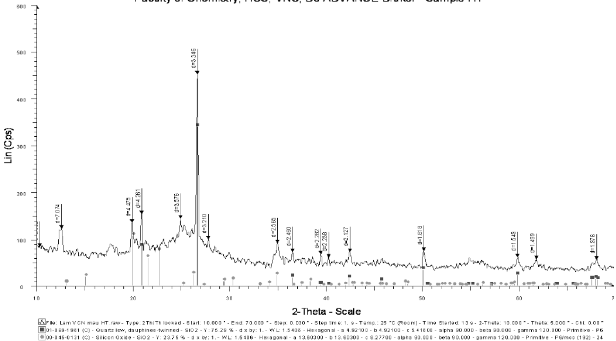
Hình 6: Giản đồ nhiễu xạ tia X của mẫu than mỏ Hồng Thái
