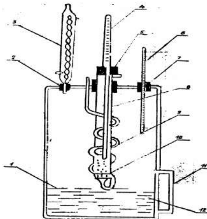
Hình 7. Thiết bị chỉ thị nhiệt
