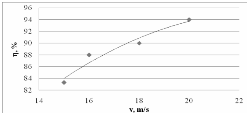
Hình 7. Hiệu quả lọc bụi theo vận tốc vào xyclon cải tiến ứng với nồng độ bụi đầu vào
