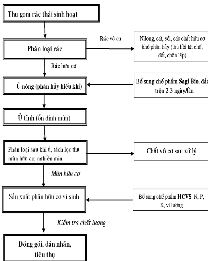
Hình 1. Quy trình xử lý và chế biến rác thải sinh hoạt thành phân hữu cơ vi sinh
