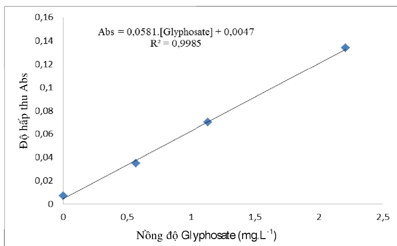
Hình 3. Đường chuẩn xác định nồng độ Glyphosate bằng phương pháp trắc quang.
