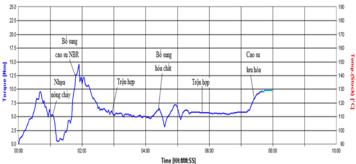
Hình 1: Biểu đồ mô men xoắn – thời gian của quá trình lưu hóa động blend NBR/PP
