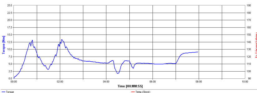
Hình 4. Biểu đồ mômen xoắn của blend NBR/PP (M3)
