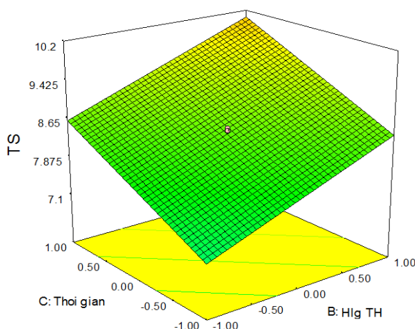
Hình 10. Mặt đáp của hai nhân tố hàm lượng chất tương hợp và thời gian
