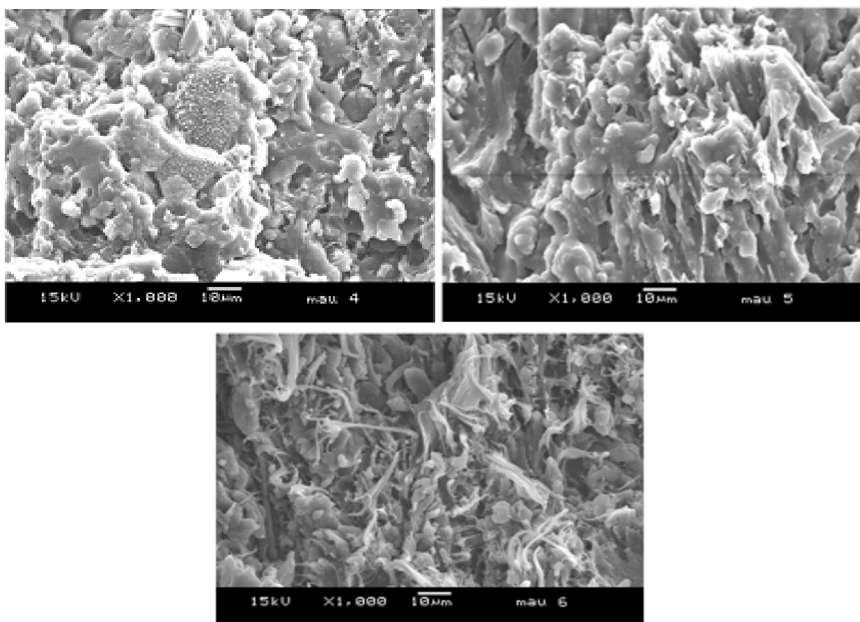
Hình 8. Ảnh chụp SEM của mẫu M4, M5, M6
