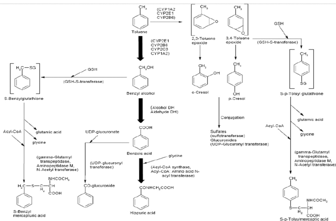
Hình 1: Sơ đồ chuyển hóa của toluen trong cơ thể người
